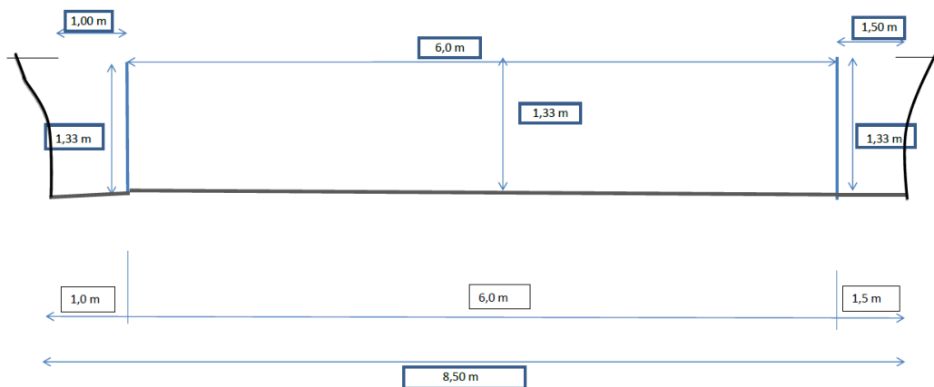
Aushubplan LÄNGSSCHNITT
